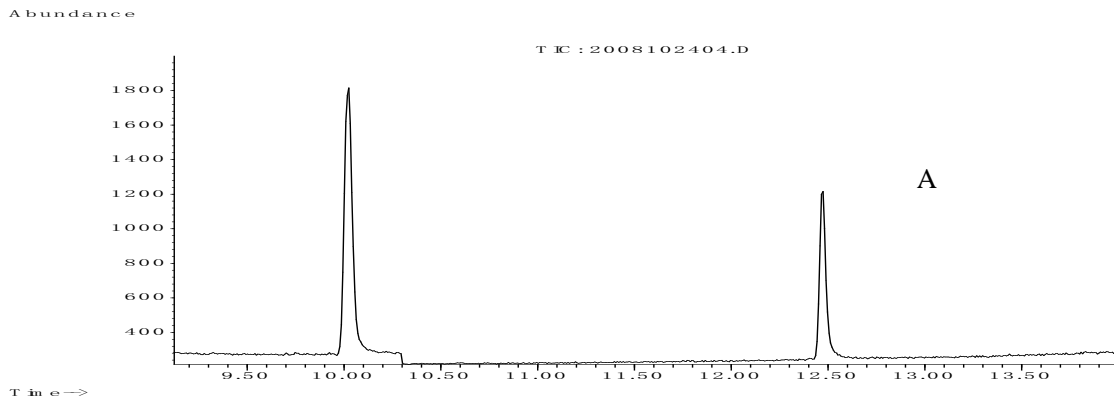
图 A 地西洋和安眠酮标准溶液选择离子色谱图 (10 \mu\text{g/L} )
