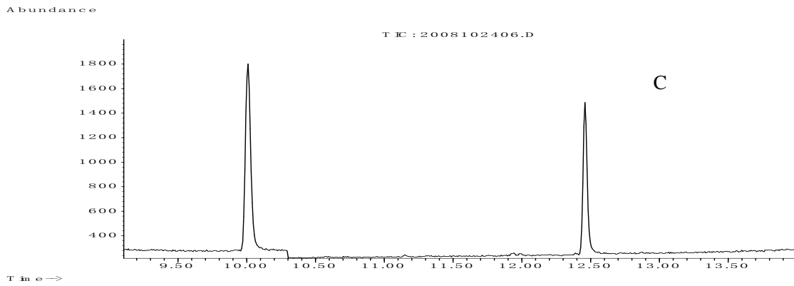
图 C 猪肌肉组织空白添加地西洋、安眠酮试样选择离子色谱图 (1 \mu\text{g/kg} )
