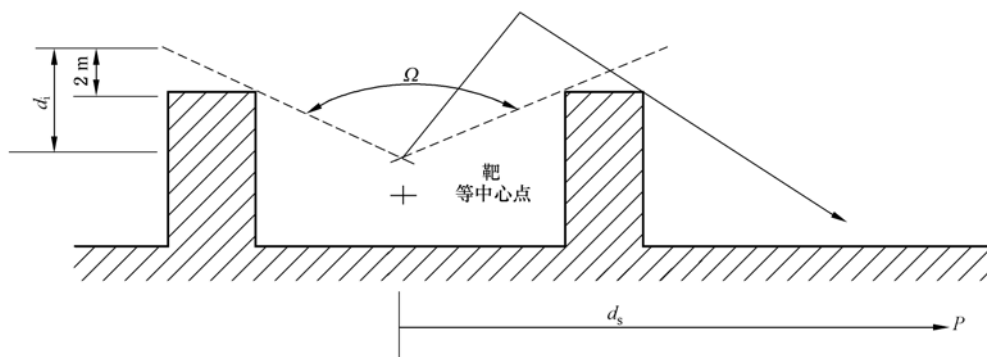
图 D.1 中子天空反散射示意图
